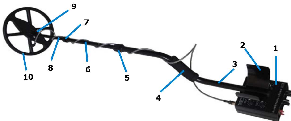
Рис.1 / Устройство металлоискателя BLISSTOOL LTC64
