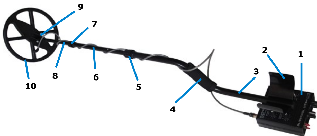
Фиг.1 / Устройство на металдетектор BLISSTOOL LTC64
